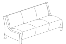
Armless Sofa W79.5" D32.75" H31.75" Seat: W71.5" D22" H19"
